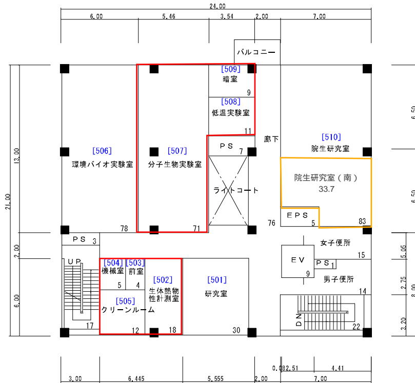
5階平面図 490㎡
