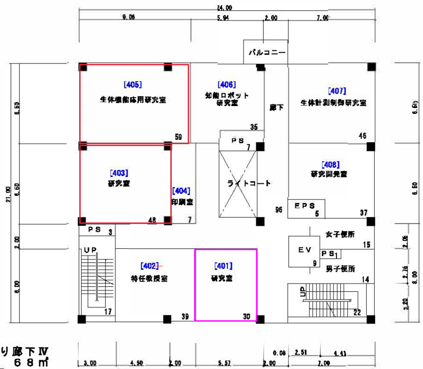
4階平面図 490㎡
